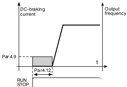
Рис. 9.10: Время торможения постоянным током при пуске
